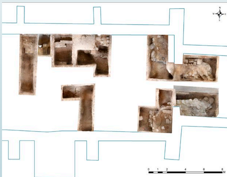
A templombelsőben kutatott szelvények a feltárt falazatokkal (fotogrammetria: Belbe Sebastian, 2022)
