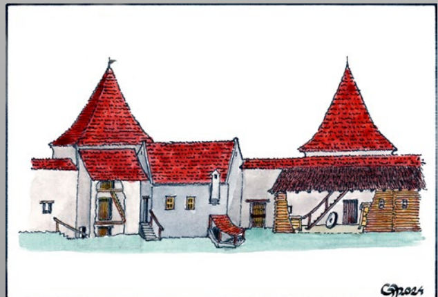
A templomvár keleti oldalának belső nézete a kéttraktusú kőépülettel és a délkeleti torony belső oldalán állt faépülettel, rekonstrukciós kísérlet, 17. század közepi állapot (a szerző adatai alapján rajzolta: Gyöngyössi János)
