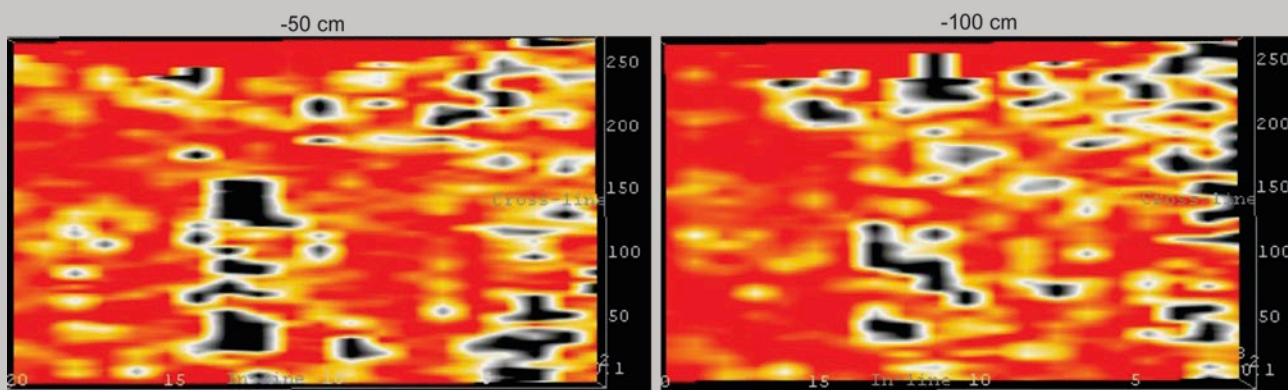
A homoródszentmártoni templomvár geofizikai kutatása – a kaputorony nyugati oldalán végzett vizsgálat színeképe -50 és -100 cm mélységekben, 2010 (készítette: Geoservice Kft.)
